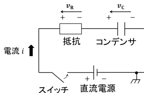
図 1 コンデンサを含む直流回路
