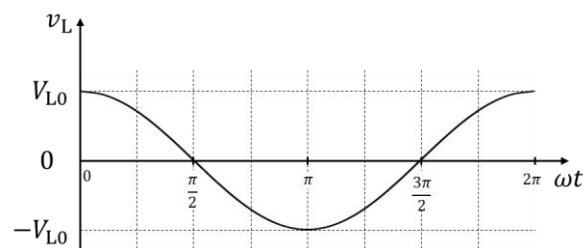
図 8 コイルにおける電圧降下の時間変化
