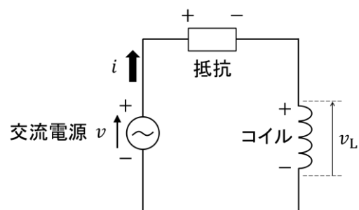
図 7 コイルを含む交流回路
