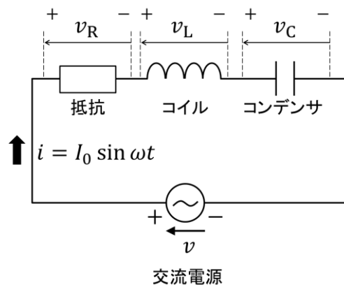
図 9 RLC 直列回路
