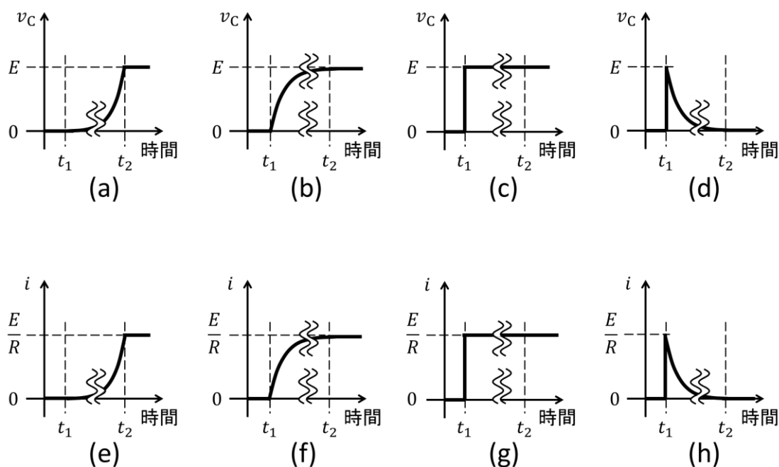
図 2 電圧降下・電流の時間変化.
