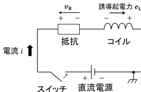
図3 コイルを含む直流回路
